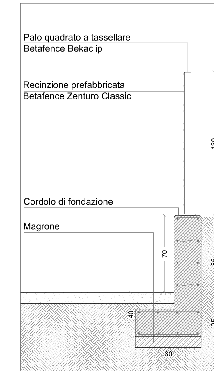
DETTAGLIO 5 - TIPO E2 Demolizione e ricostruzione recinzione con sbancamento di terreno verso Via Gemina
