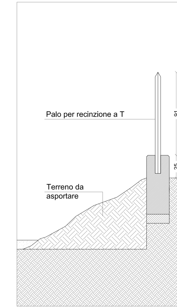
DETTAGLIO - TIPO E2 Stato di fatto recinzione
