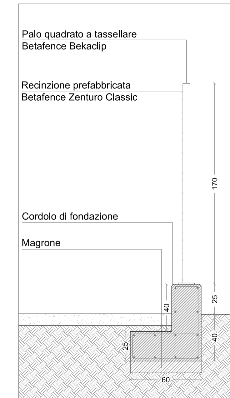
DETTAGLIO 5 - TIPO E1 Demolizione e ricostruzione recinzione
