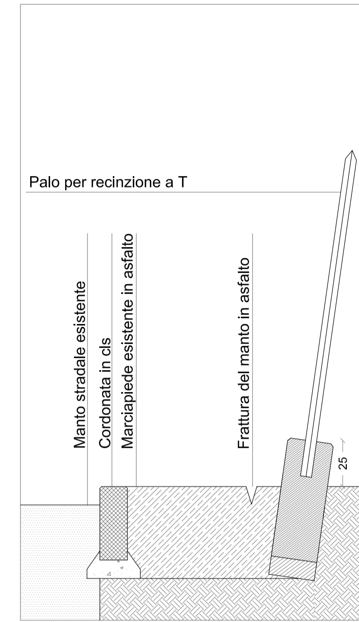
DETTAGLIO - TIPO B Stato di fatto recinzione
