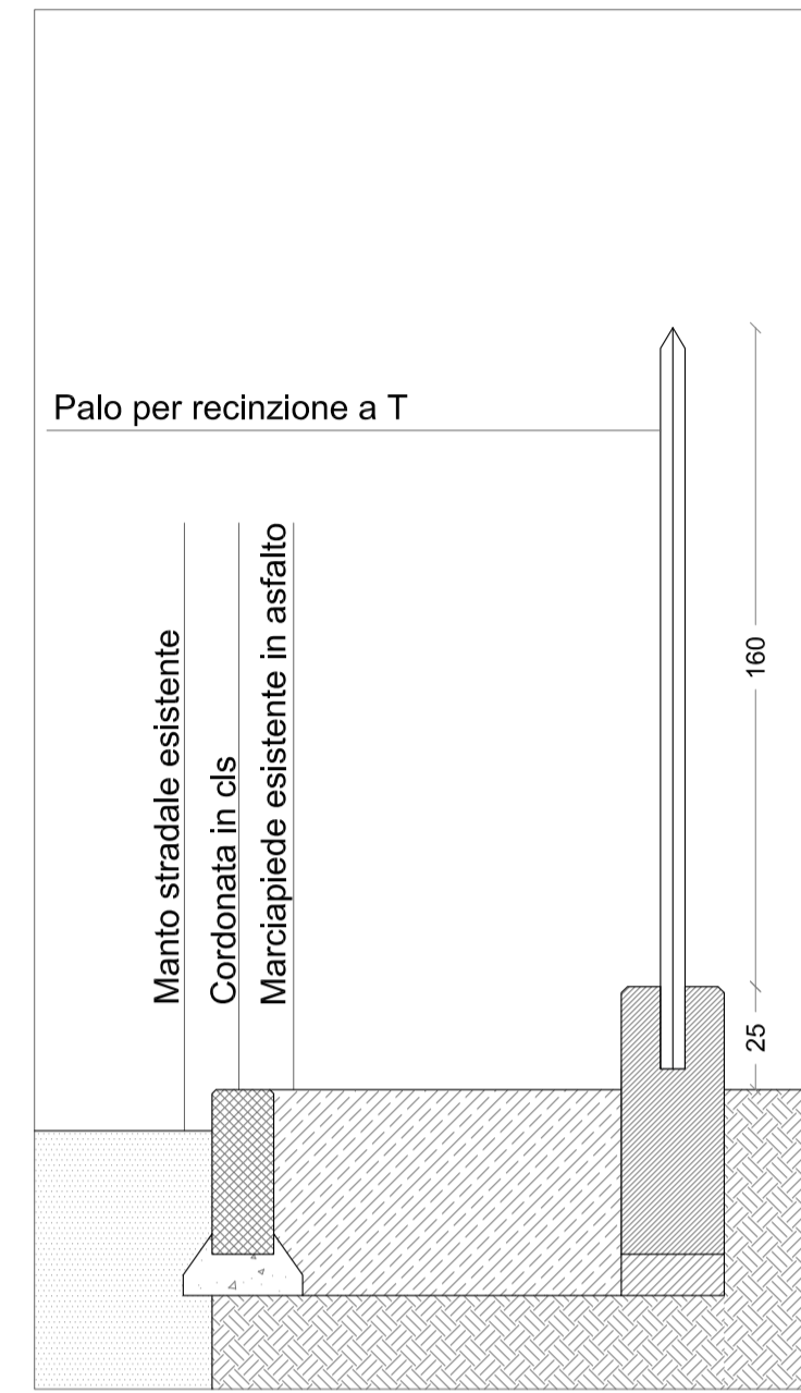
DETTAGLIO - TIPO A e TIPO D Stato di fatto recinzione
