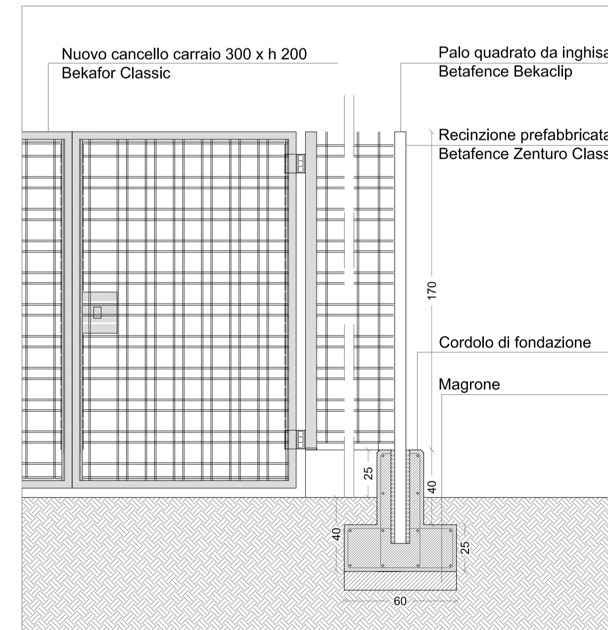
DETTAGLIO 3 - TIPO C Recinzione fondazione eretta e sostituzione cancello
