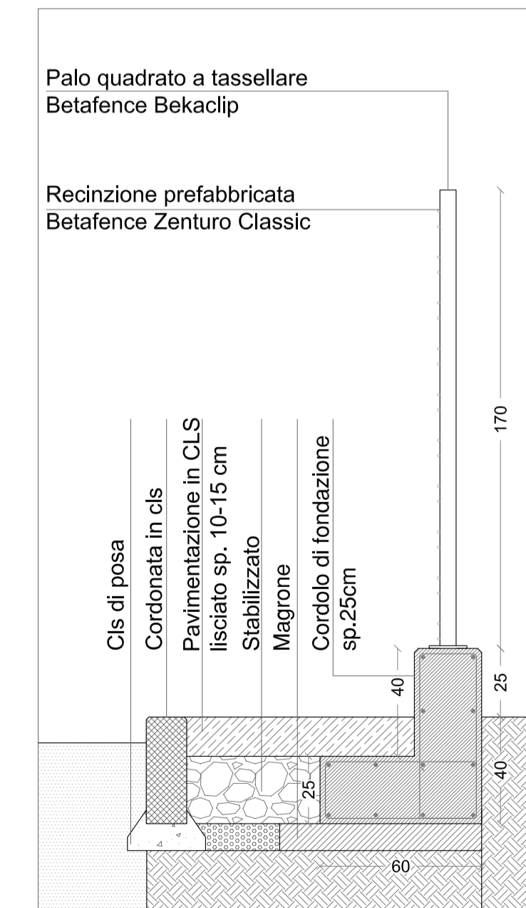
DETTAGLIO 4 - TIPO D Nuova recinzione e ricostruzione marciapiede
