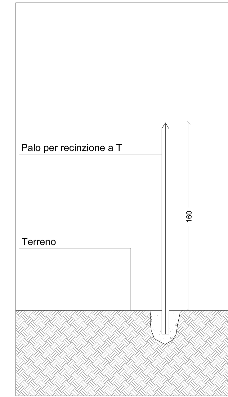
DETTAGLIO - TIPO C Stato di fatto recinzione
