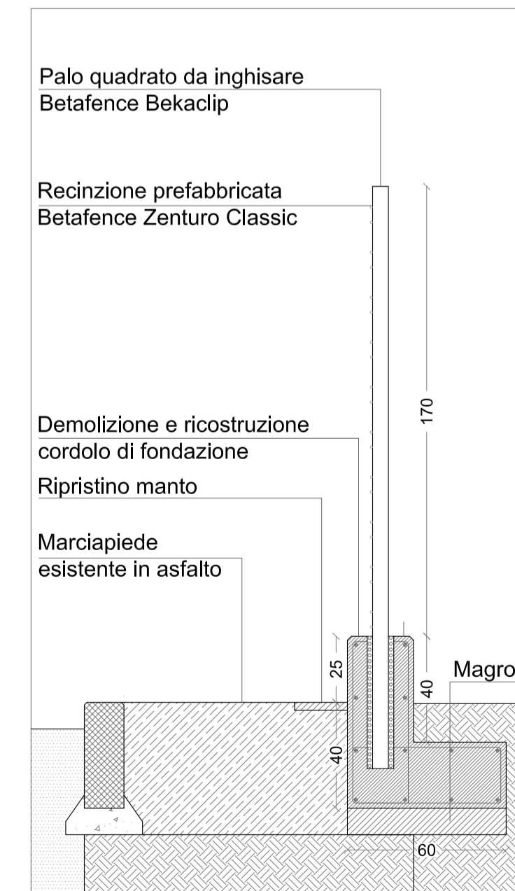
DETTAGLIO 2 - TIPO B Demolizione e ricostruzione recinzione e cordolo di fondazione
