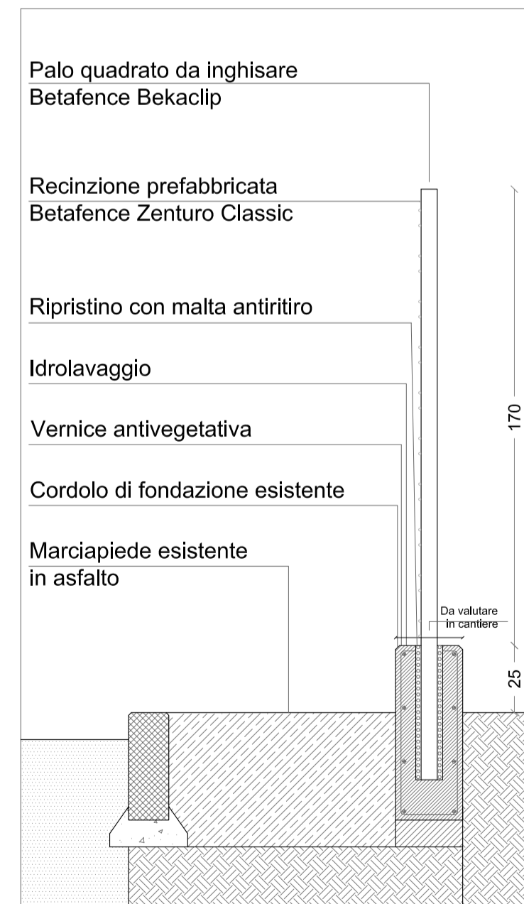
DETTAGLIO 1 - TIPO A Sostituzione rete
