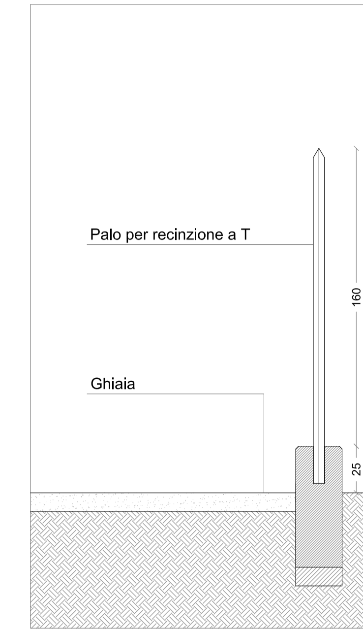
DETTAGLIO - TIPO E1 Stato di fatto recinzione
